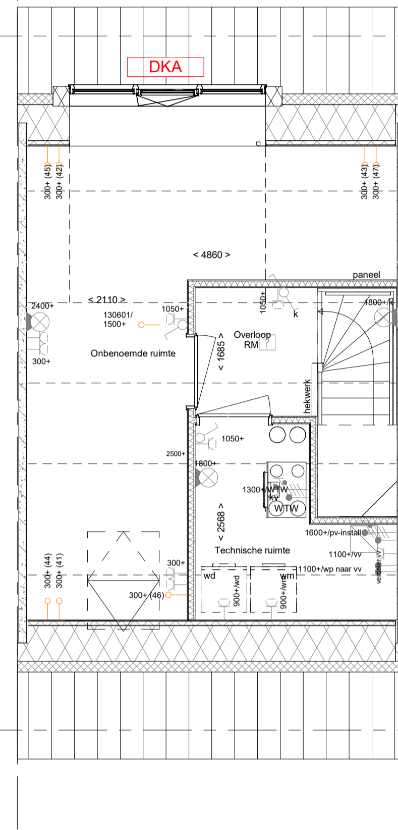
PL0202 - Plattegrond 2e verdieping met overloop, technische ruimte en 1 onbenoemde ruimte. DKA302 - Dakkapel achtergevel met verjongde overstek
