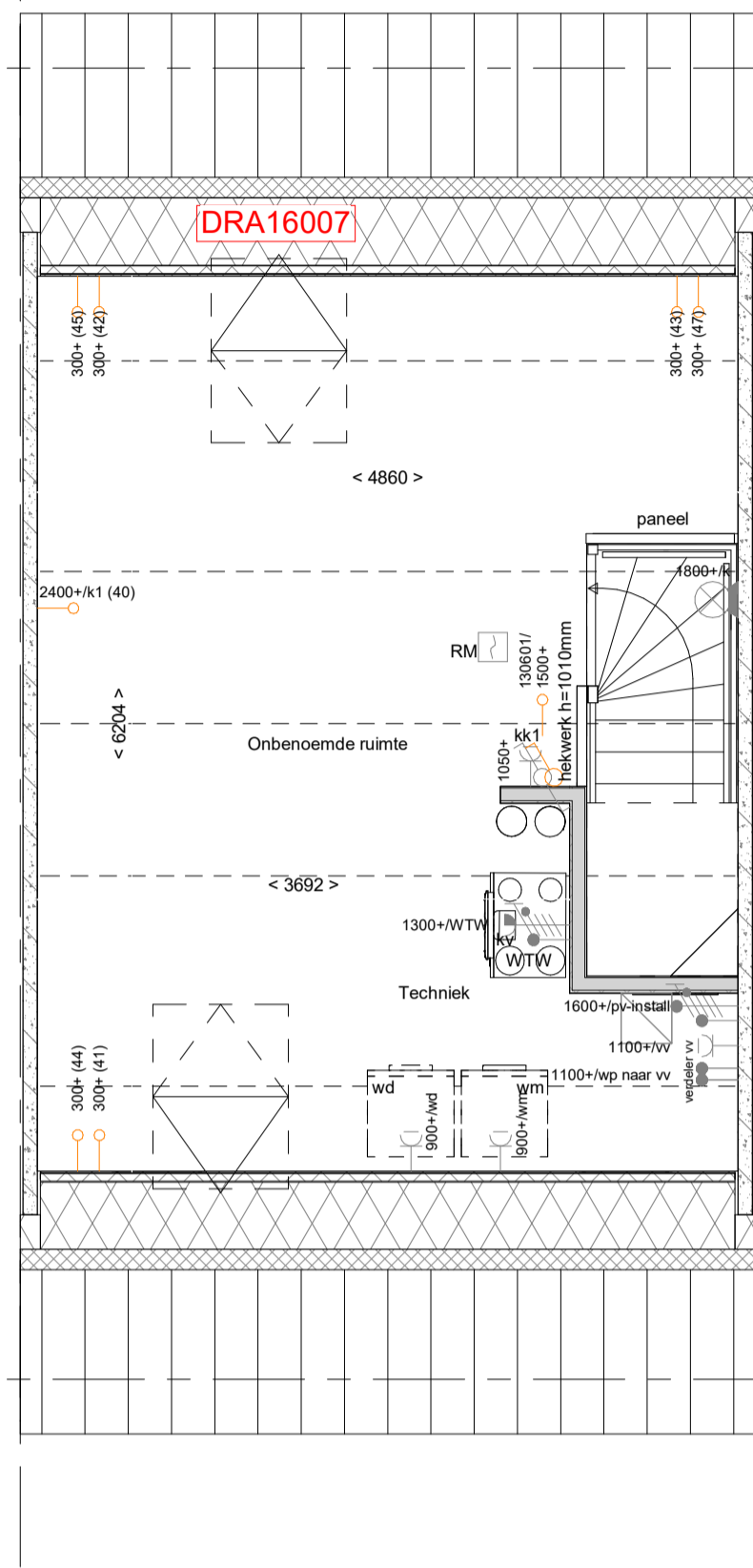
DRA16007 - Dakraam in de achtergevel t.p.v. de onbenoemde ruimte
