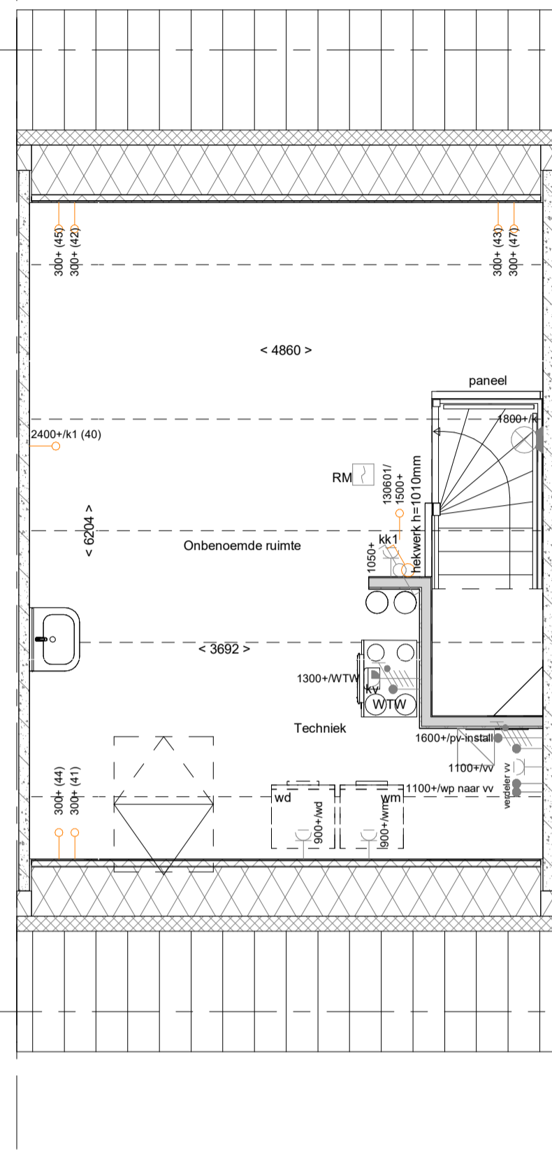
PL0201 - Plattegrond 2e verdieping in basis uitvoering 311320xxx - Aanbrengen wastafelcombinatie op 2e verdieping
