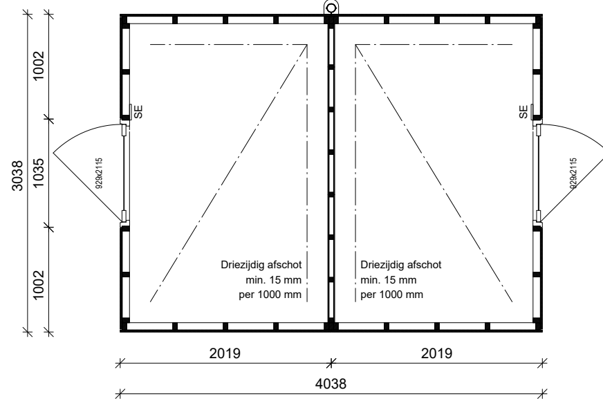
PLATTEGROND (Tuinzijde)
