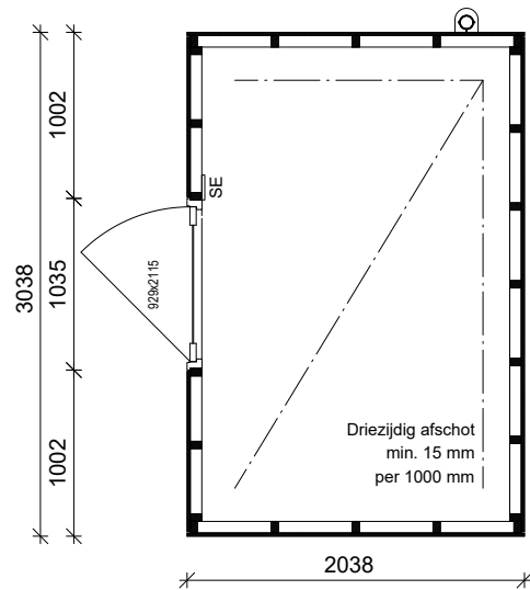
PLATTEGROND (Tuinzijde)
